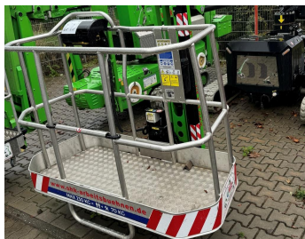
JIBBI 1670, ALM-002319-Drehbahrer Arbeitskorb
